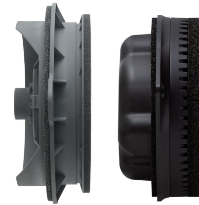
ユニット背面が開放されエンクロージャ機能のない一般的な純正16cmスピーカー(概念説明用モデル) 専用開発の高性能ユニットとエンクロージャを一体化したSonicPLUSスピーカーモジュール
