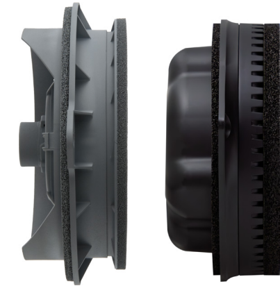
ユニット背面が解放されエンクロージャ機能のない一般的な純正16cmスピーカー (概念説明用モデル) 専用開発の高性能ユニットとエンクロージャを一体化したSonicPLUSスピーカーモジュール
