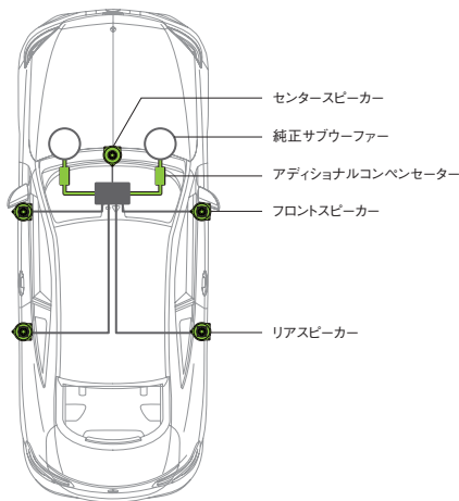
SC-C205Mn 5スピーカーモジュール システム構成図
