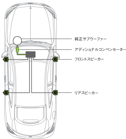
SC-C205M 4スピーカーモジュール システム構成図
