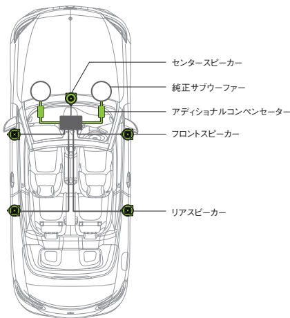
SC-A205Mn 5スピーカーモジュール システム構成図
