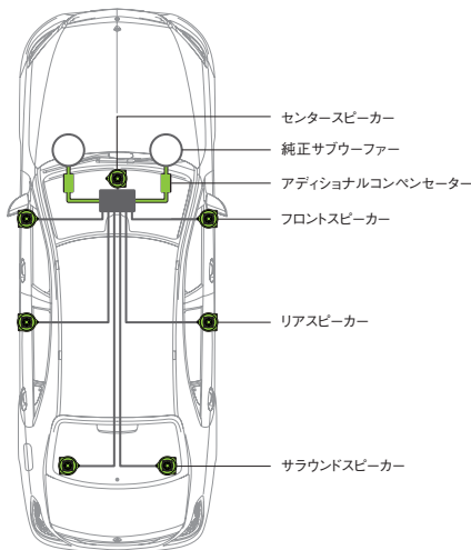
SC-222M 7スピーカーモジュール システム構成図
