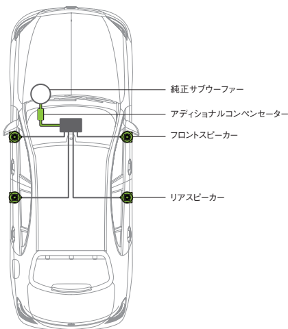
SC-213M 4スピーカーモジュール システム構成図
