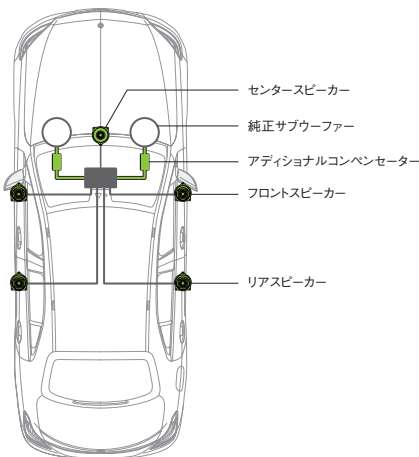
SC-205Mn 5スピーカーモジュール システム構成図
