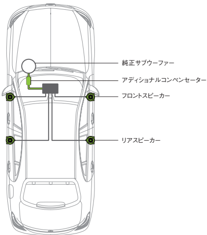
SC-213M 4スピーカーモジュール システム構成図 (セダン)
