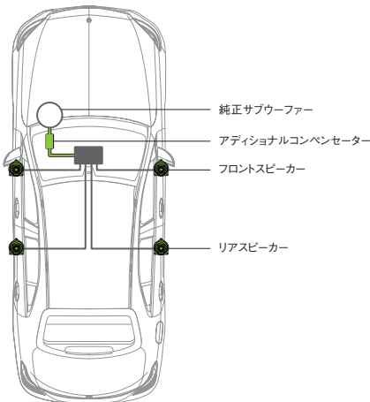
SC-205M 4スピーカーモジュール システム構成図
